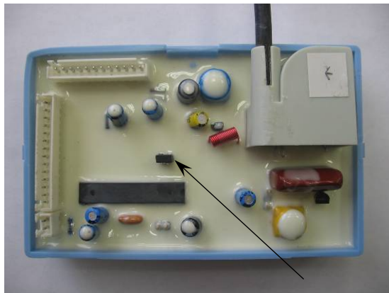
Рисунок 9. Место установки переключки в блоке управления электронном
